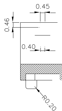
A-A' Section
